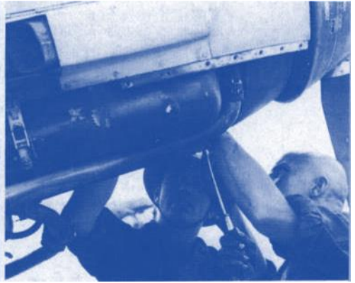
Nächtlicher Motorwechsel im Werkzelt in der Wüste (oben rechts)
