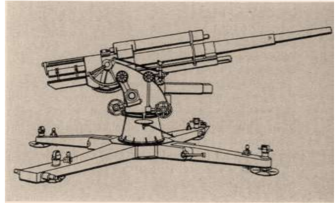
Oben: Deutsche Fliegerabwehrkanone 8,8-cm-Flak/18, gleichzeitig das gefürchtetste Panzerabwehrgeschütz des Krieges (ab 1937)
