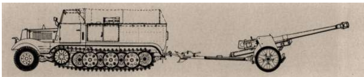
Deutsche Panzerjägerkanone 7,5 cm 40 mit leichtem Zugkraftwagen 3 t (Sd Kfz 11)
