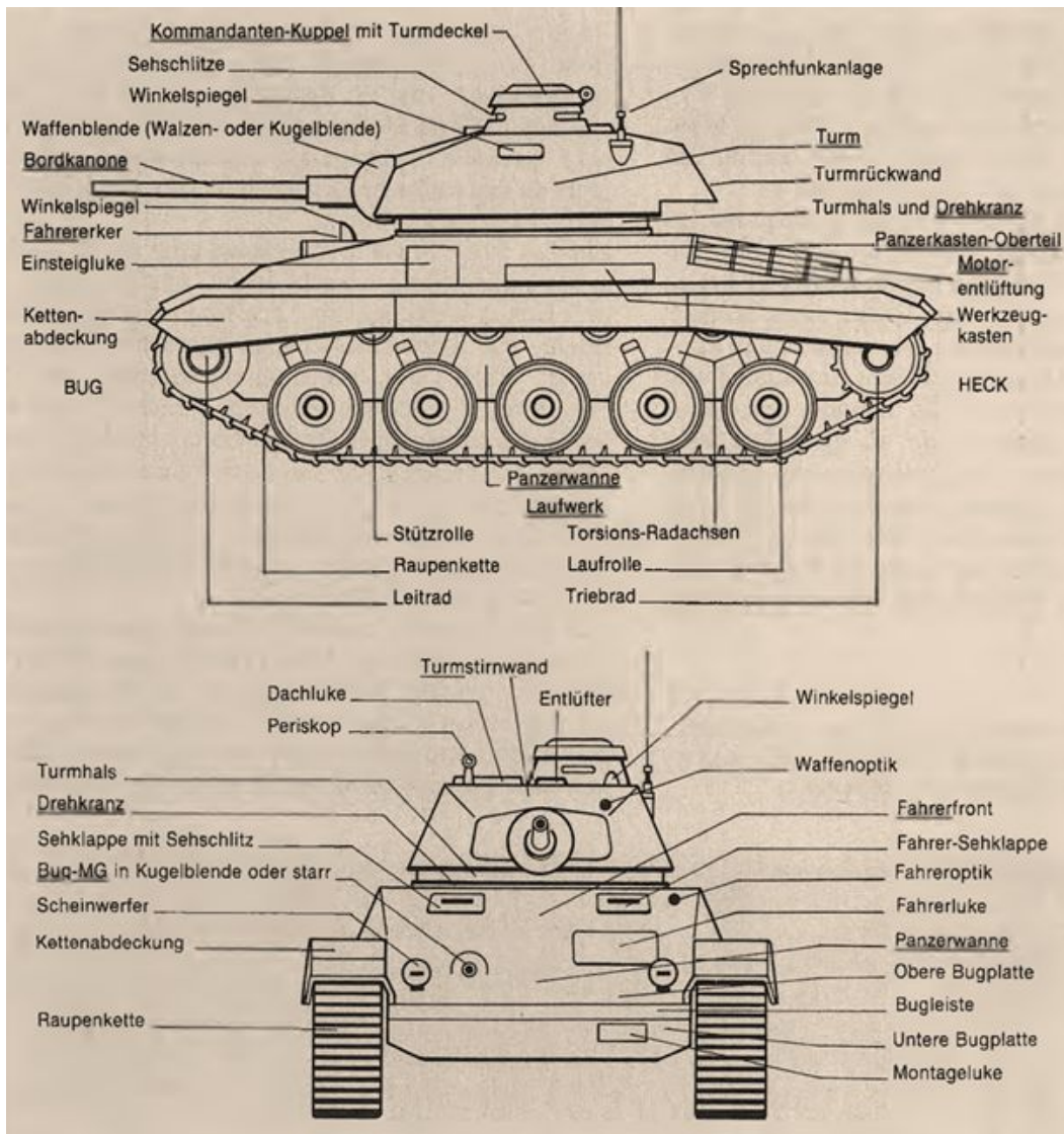
Schema eines Panzers
