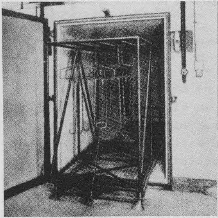
Abb. 27 Transportwagen zur Aufnahme von etwa 15 Monturen. Zwei solcher Wagen könnten hintereinander in eine Zelle geschoben werden, um die 10 cbm zu füllen.
