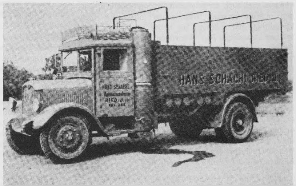
Abb. 1. Saurer 5 BHw. mit Holzgasantrieb.
