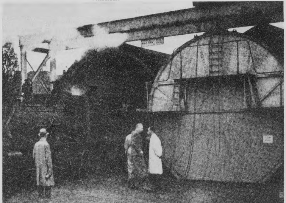
41. Vakuum-Eisenbahnbegasungsanlage — verlauste Wagen werden eingefahren.
