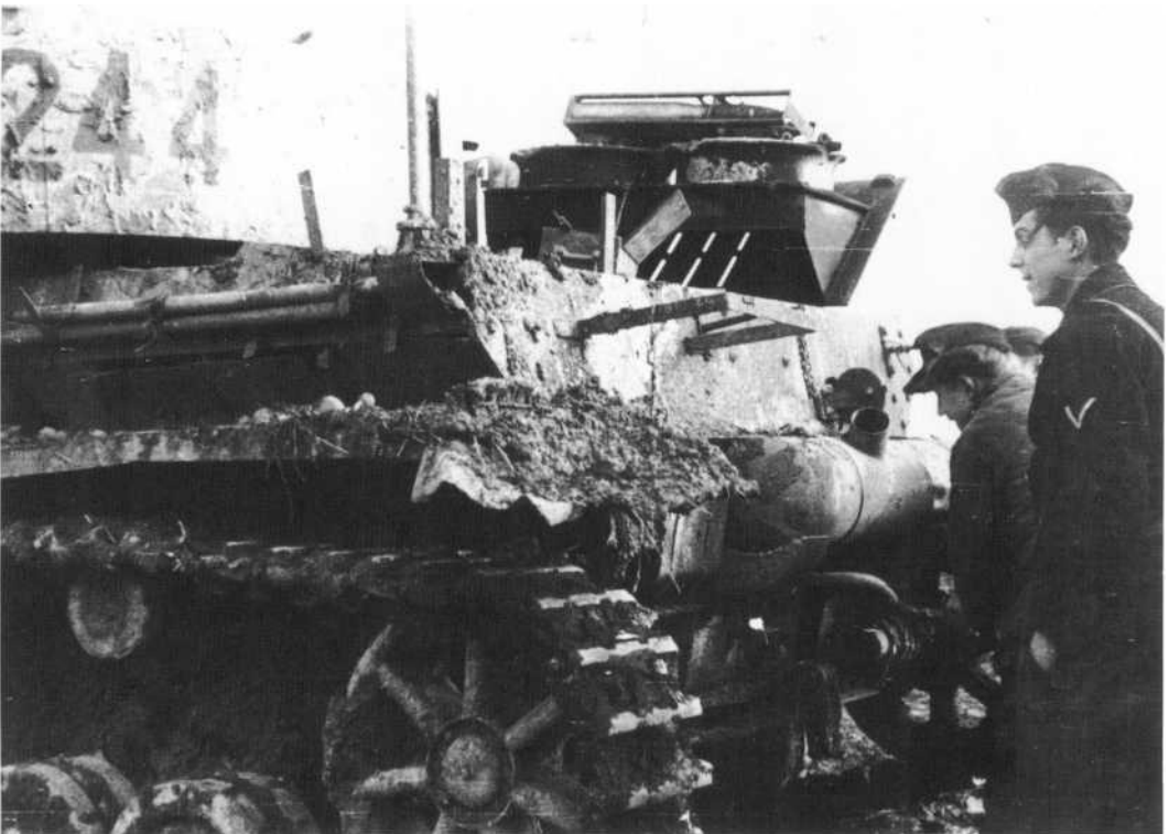
Ständige Reparaturarbeiten am Panzer: Fahrer und Kommandant spannen beim Pz. 1244 die Ketten nach. Die gepanzerte Motorabdeckplatte mit Kühlergrill und Luftgebläse sind aufgeklappt. Auf dem Gebläse sind zwei Panzergranaten in einem Holzgestell abgelegt. Der Pz. ist deutlich von der Schwarzerde in der Ukraine gezeichnet.
