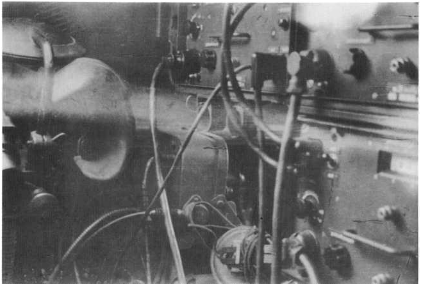
Der Funkerplatz: Ein Sender und zwei Empfänger in einem Gestell über dem Getriebe. Rechts der Griff des MG 42 mit Gummiblende, Zieloptik und Kopfstütze.
