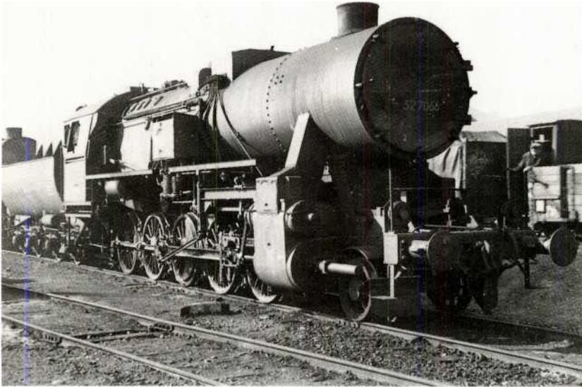
Dampflokomotiven für den Transport nach Russland: Deutsche Kriegslok 527066 bei einer Fahrt durch Österreich.
